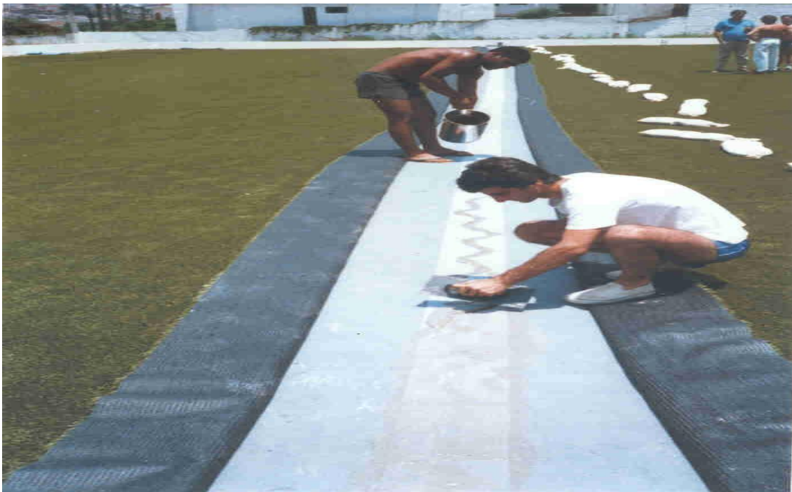
Foto 4 – União das placas da grama artificial através da colagem com fita de PVC.
