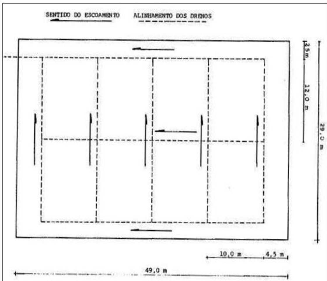
Figura 1 – Esquema do sistema de valas drenantes (sem escala).
